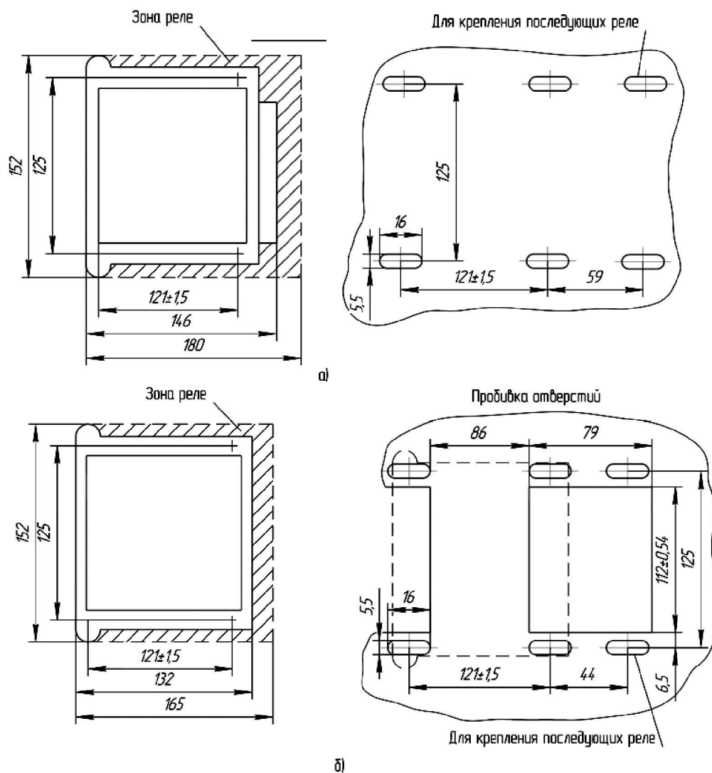
Рисунок 4 – Зона реле и пробивка отверстий под установку
